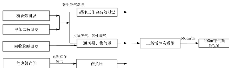
图 4-1 本项目主要废气收集和处理措施流程示意图
