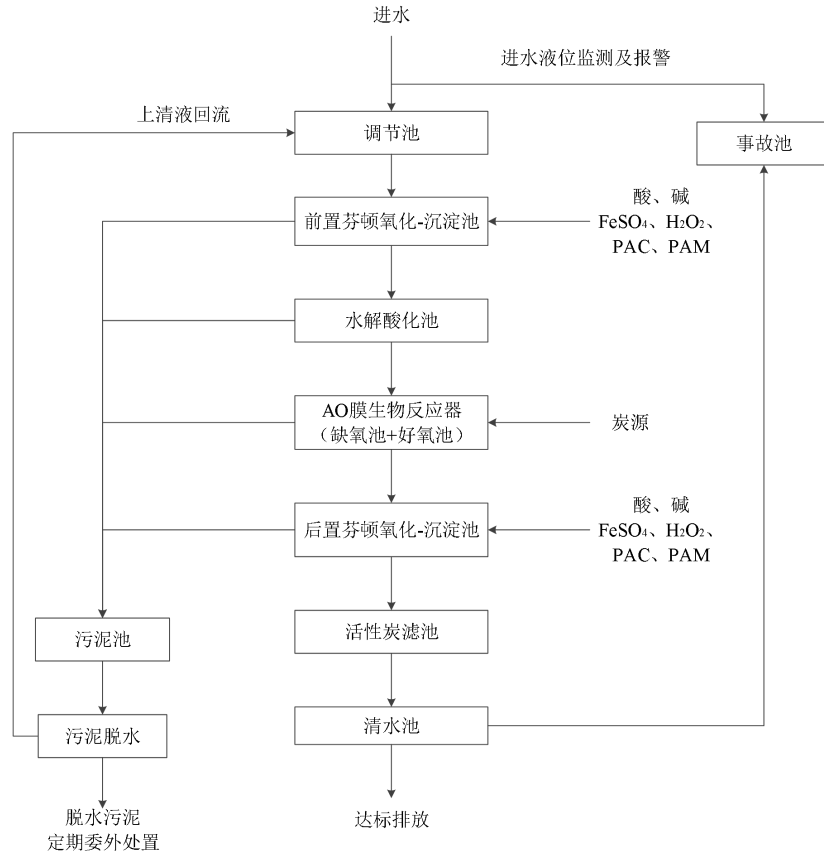
图 4-3 中丹园一期实验废水处理站工艺流程示意图
