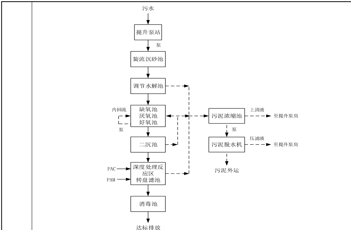
图 4-4 盘城污水处理厂工艺流程图
