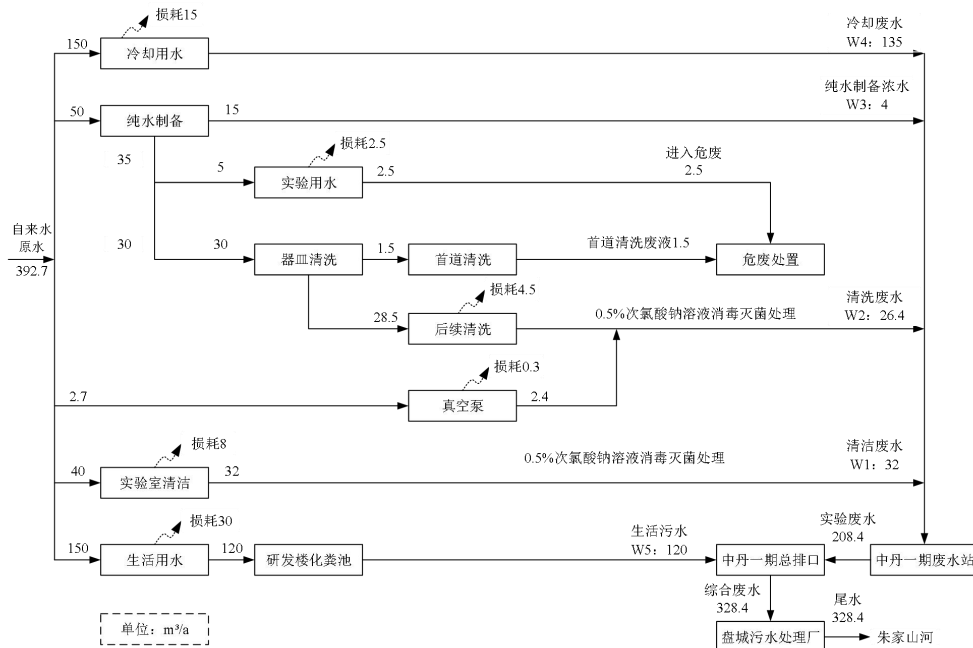
图 4-2 项目水平衡图
