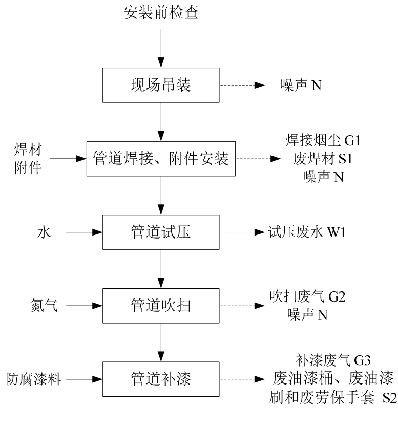
图 2-1 施工工艺及排污流程图
