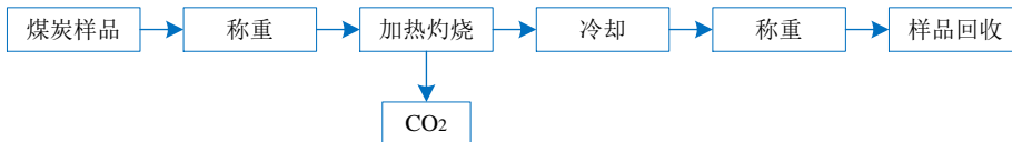
图 2-9 煤炭灰分分析工艺流程及产排污环节图
