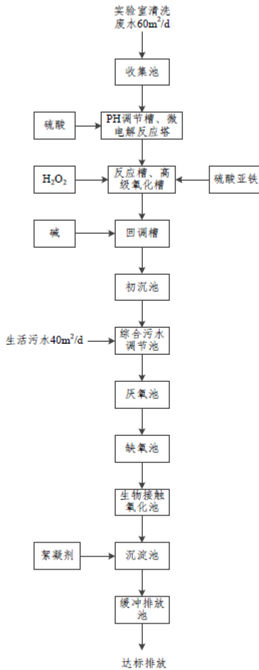
图4-2 C-Park 综合服务区污水预处理工艺流程 废水处理站各处理单元处理效果见下表。
