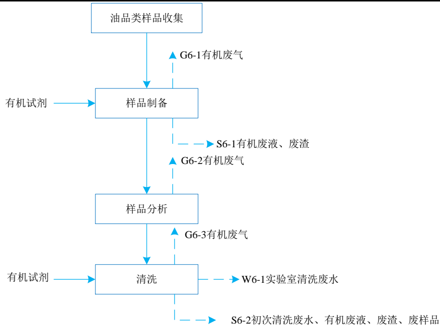
图 2-7 油品类样品检测工艺流程及产排污环节图
