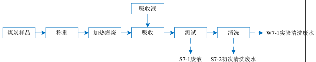
图 2-10 煤炭全硫含量分析工艺流程及产排污环节图
