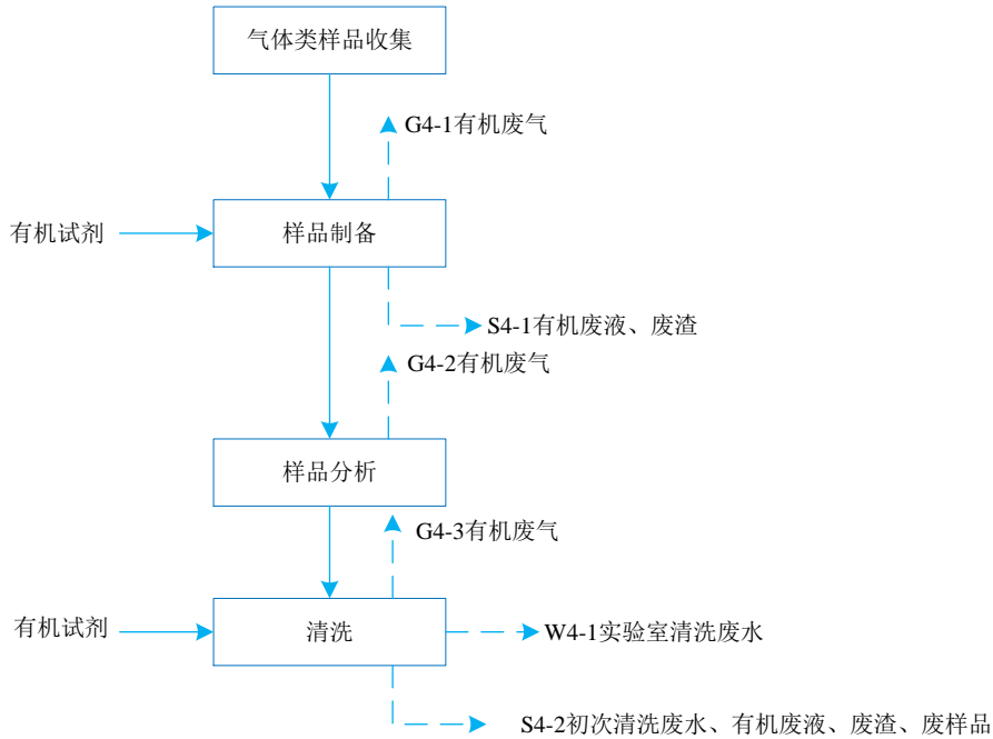
图 2-5 气体类样品检测工艺流程及产排污环节图
