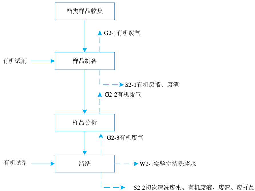
图 2-3 酯类样品检测工艺流程及产排污环节图
