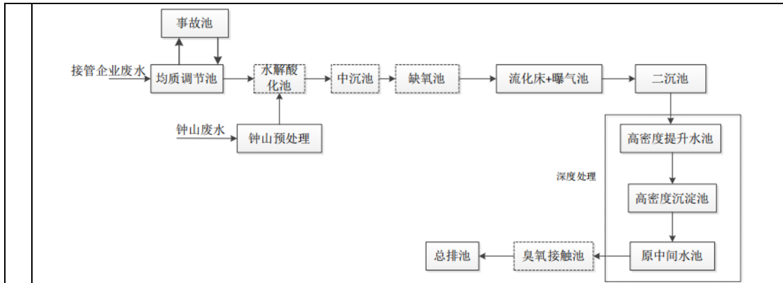
图4-3 南京胜科水务有限公司一期工艺流程图
