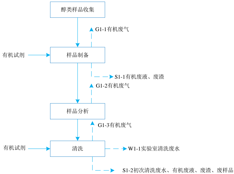
图 2-2 醇类样品检测工艺流程及产排污环节图
