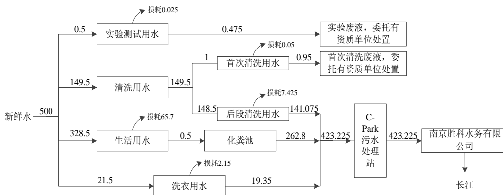
图 4-1 本项目水平衡图 (单位: m³/a)
